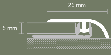
END-PROFILE PERFIL DE ACABADO
