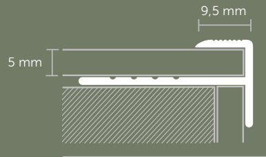
STEP PROFILE PERFIL DE PELDAÑO
