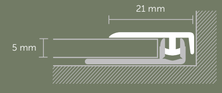
END-PROFILE WALL PERFIL DE ACABADO PARED
