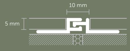
DILATATION PROFILE PERFIL DE DILATACIÓN
