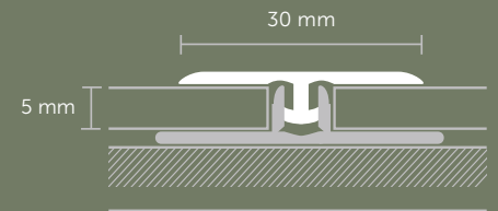
TRANSITION PROFILE PERFIL DE TRANSICIÓN
